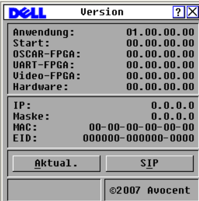
Abbildung 3-11. Dialogfeld „Version“
