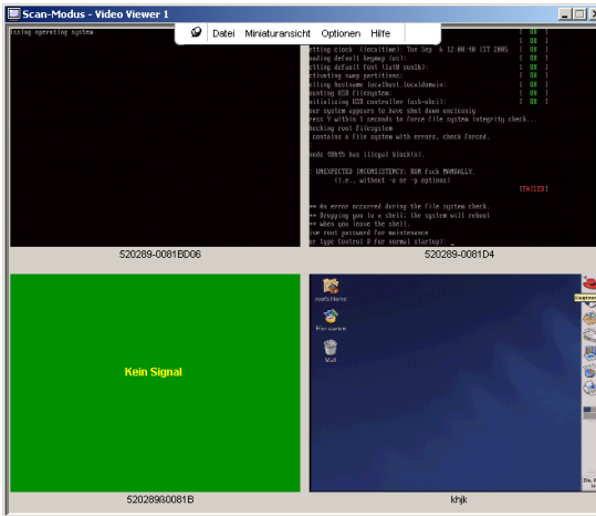
Abbildung 4-9. Viewer – Miniaturansichten
