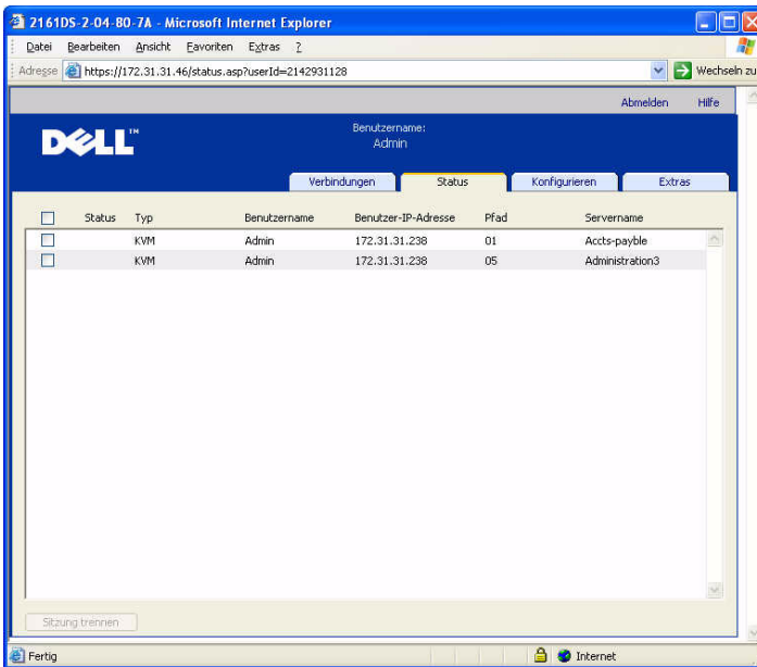
Abbildung 6-17. Fenster „Benutzerstatus“
